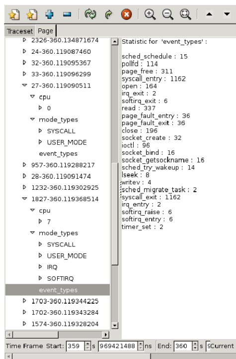
Figure 3.2 Statistiques de LTTV groupées par processus
